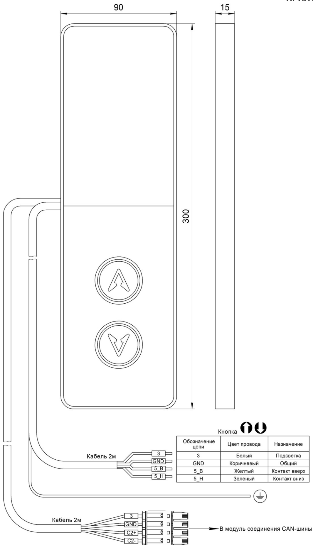
Рис.1 Внешний вид Вызывной пост ОНИКС НШЕК.468381.022
